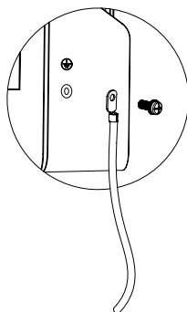
Abbildung 5-8 Anschluss der Erdungsklemme
