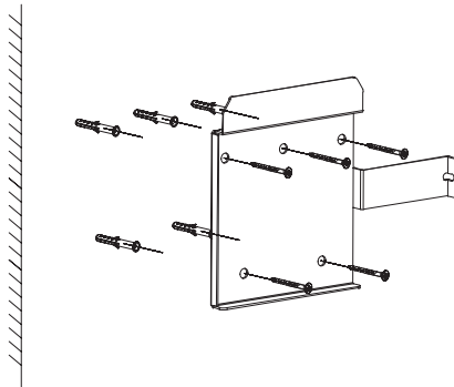
Abbildung 5-6 Befestigung der Wandhalterung
