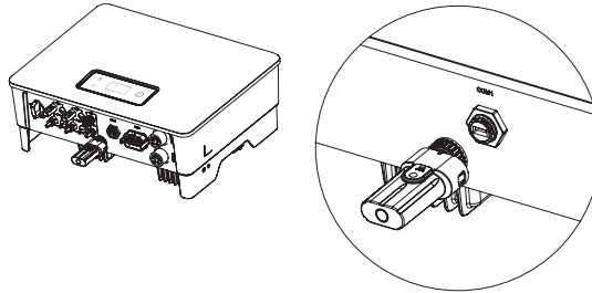
Abbildung 6-10 Installation des Überwachungsgeräts
