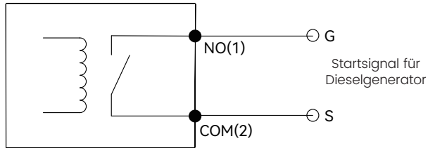
Wechselrichter-Multifunktionsrelais
