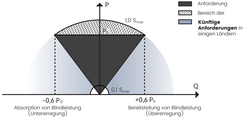
Abbildung 8-1 Leistungsvermögen
