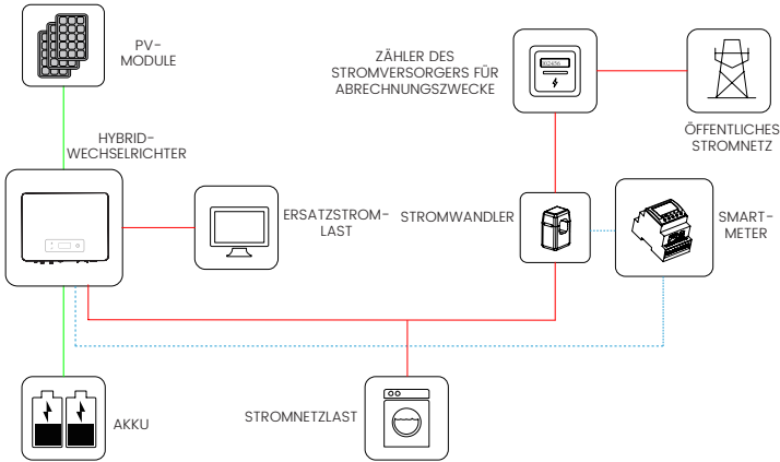
Abbildung 4-1 Schematische Darstellung des Hybridsystems
