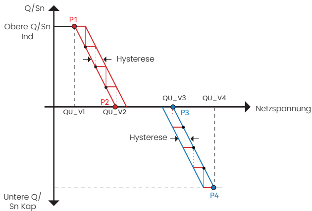
Abbildung 8-3 Q(U)-Kurve
