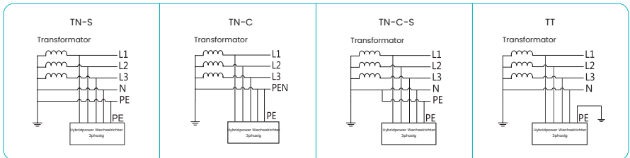
Abbildung 4-2 Anwendbare Stromnetztypen
