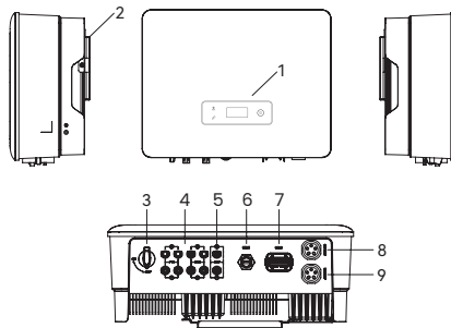
Abbildung 4-3 Aussehen des Wechselrichters
