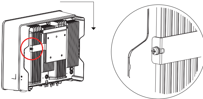
Abbildung 5-7 Montage des Wechselrichters
