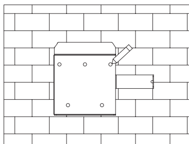
Abbildung 5-5 Markierung der Bohrungspositionen mit Wandhalterung
