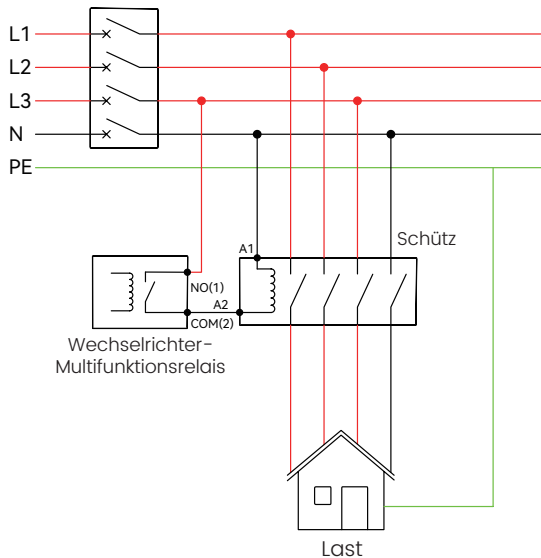
Abbildung 6-25 Anschlussschema Laststeuerung
