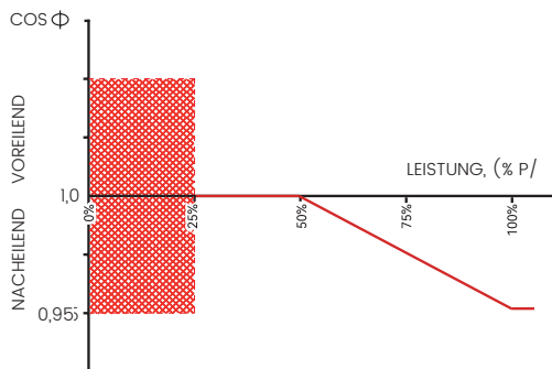
Abbildung 8-2 Q(P)-Kurve
