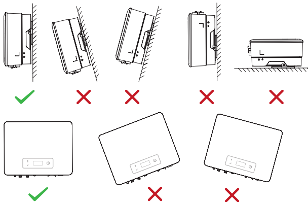
Abbildung 5-3 Zulässige und unzulässige Montagepositionen
