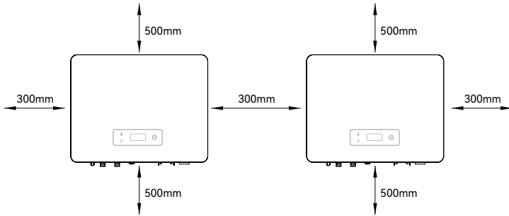
Abbildung 5-2 Empfohlener Installationsabstand
