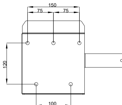
Abbildung 5-4 Abmessungen der Wandhalterung
