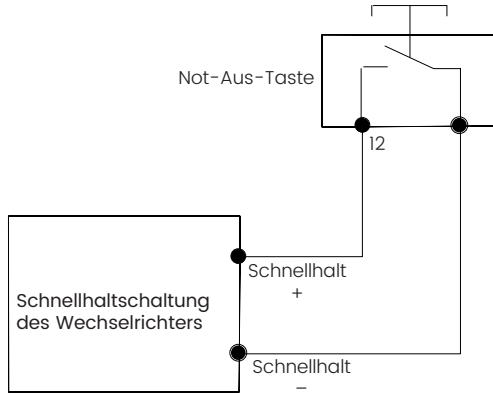
Abbildung 6-28 Anschlusschema des Schnellhalts
